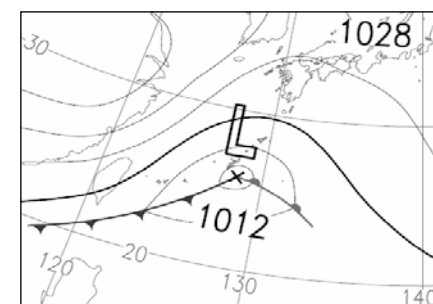
地上天気図 2005年3月3日9時
